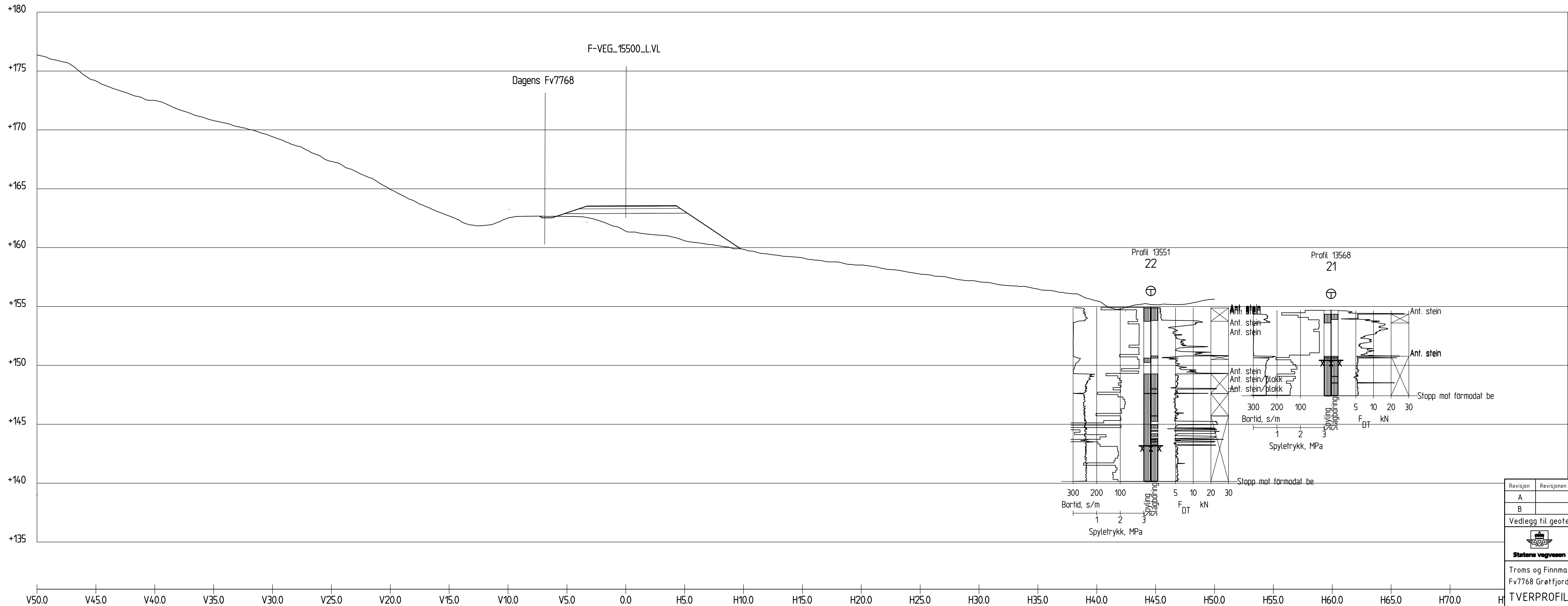
Profil 13560 1 : 200
