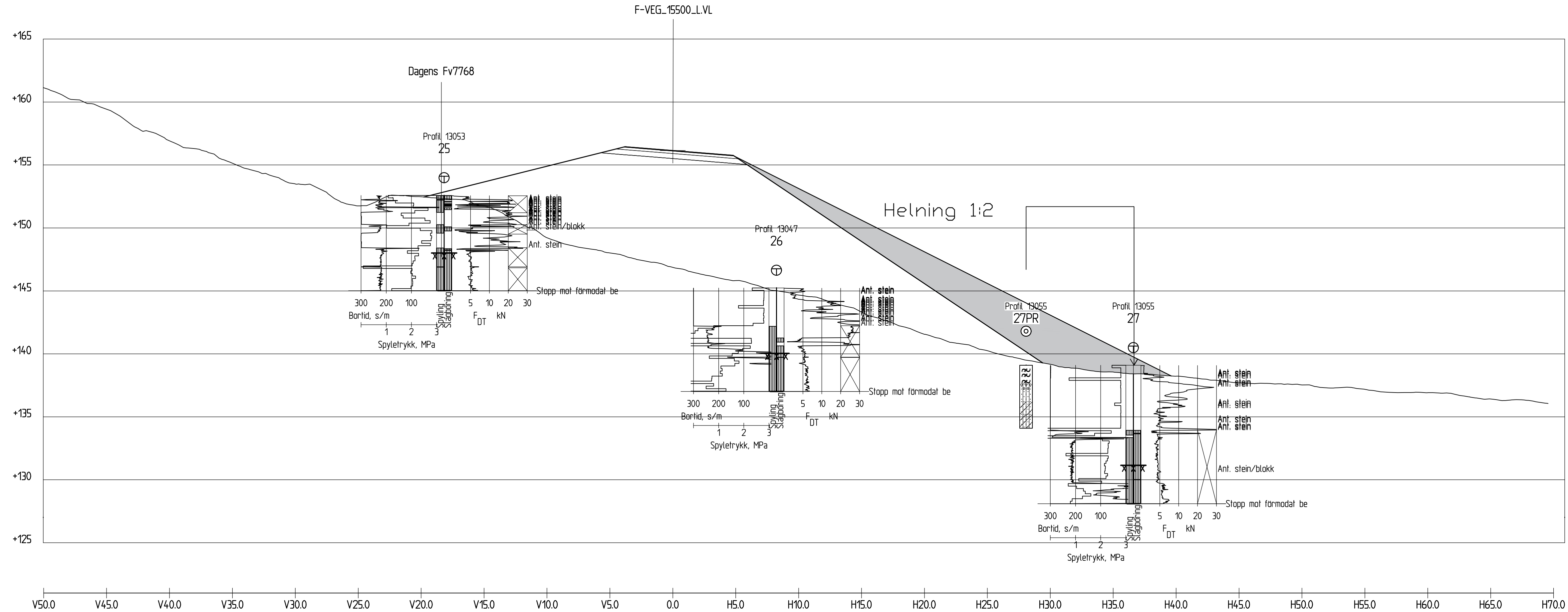
Profil 13050 1 : 200
