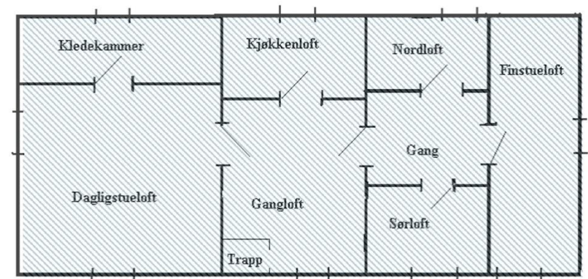
Grunnplan 2. etasje
