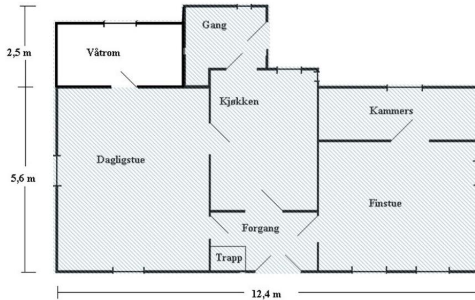
Grunnplan 1. etasje
